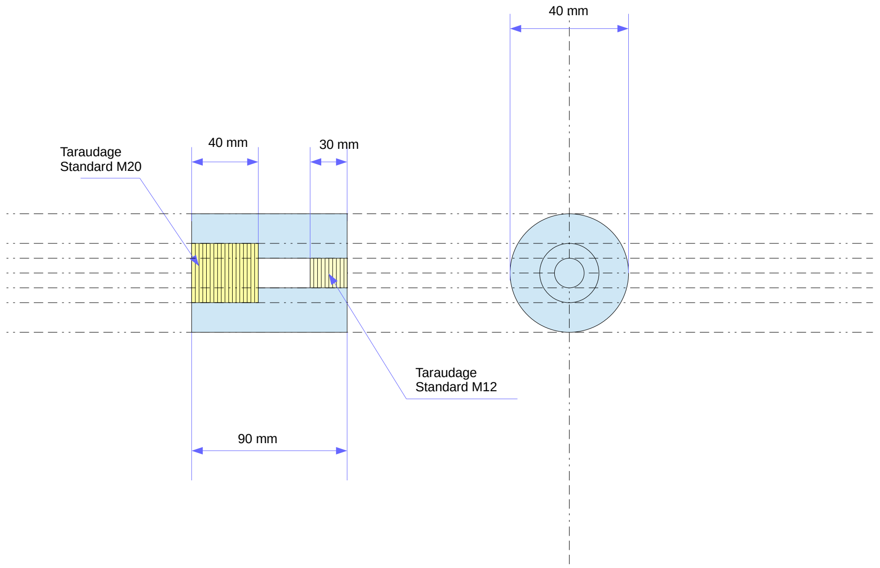
Projet 3 : Adaptateur de montage Moteur SNR
