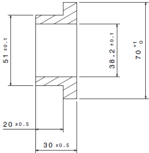
Coupe A-A Echelle : 1:1
