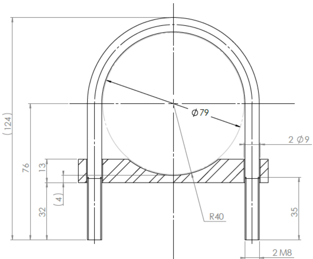
COUPE A-A
