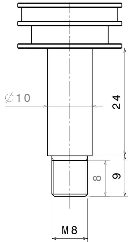
Vue de face Echelle : 2:1
