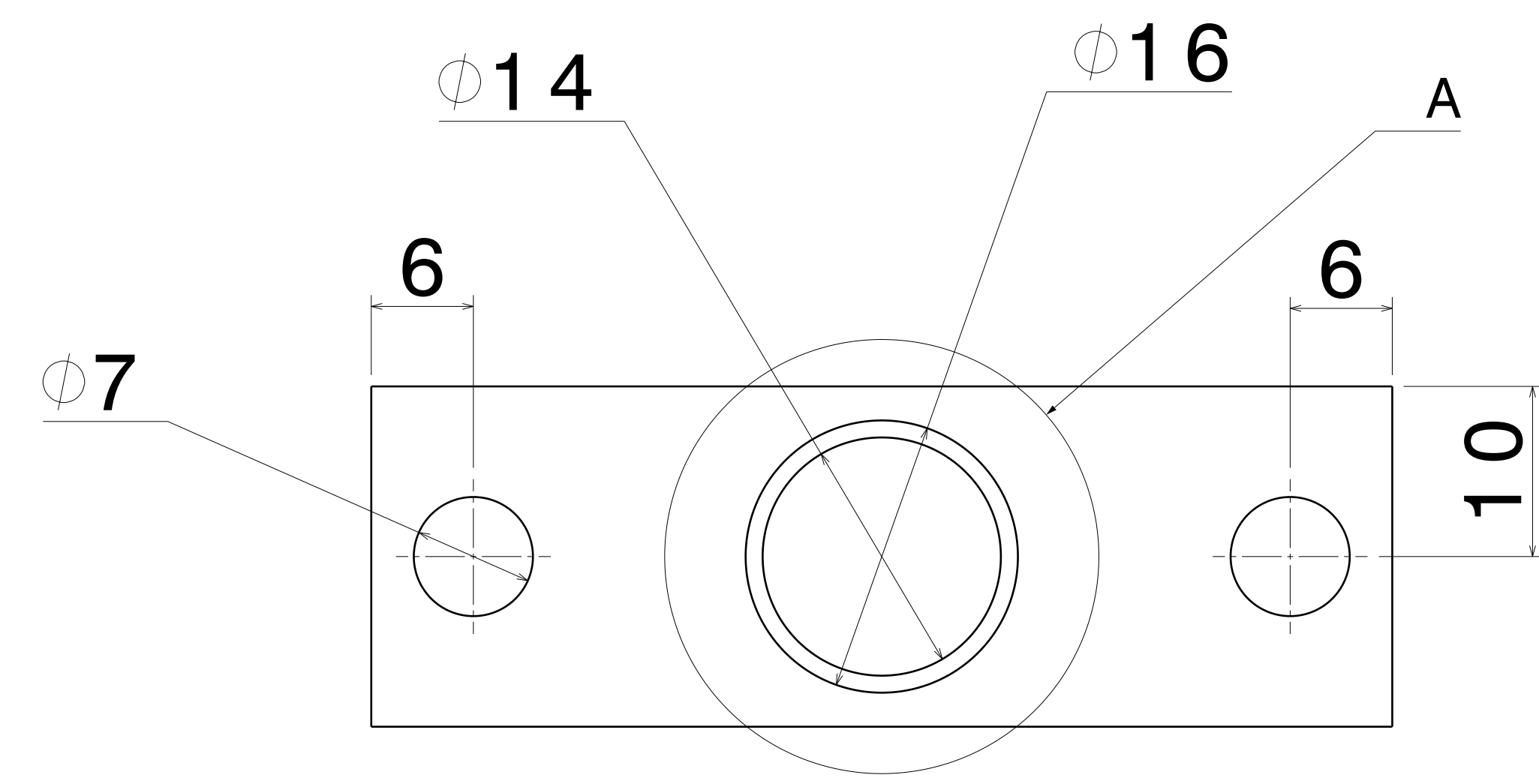
Vue de dessous Echelle : 3:1
