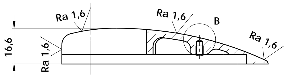
COUPE A-A
