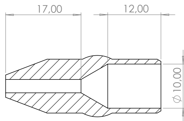
COUPE A-A
