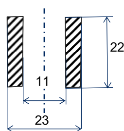
Entretoise 23
