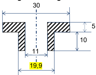
Bague blocage 20
