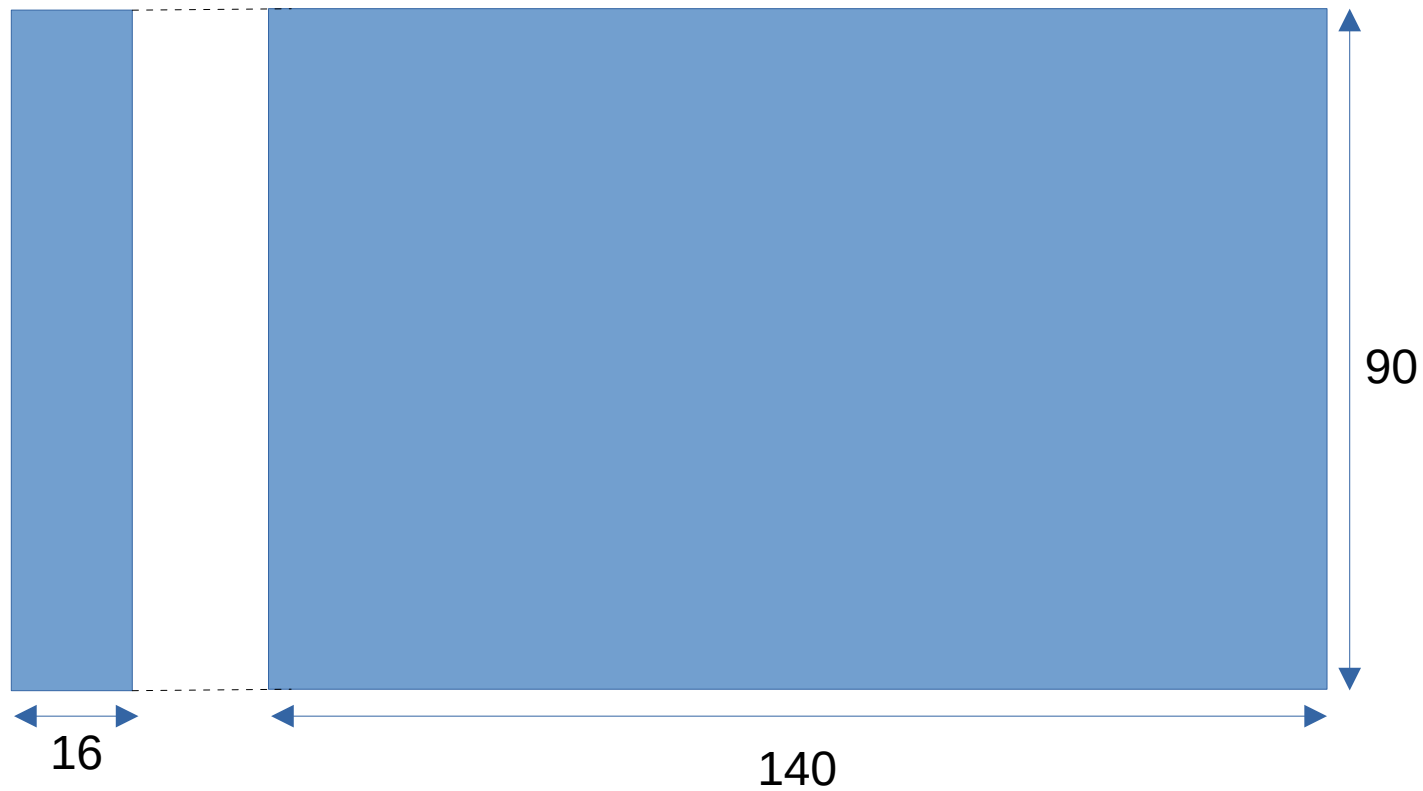
Plat 140mm x 90mm x 16mm Matériaux acier ou fer ou laiton
