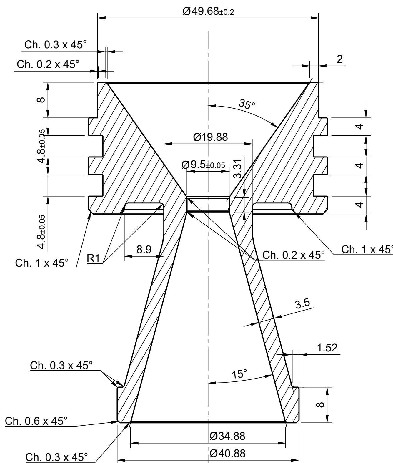
A-A (2:1)
