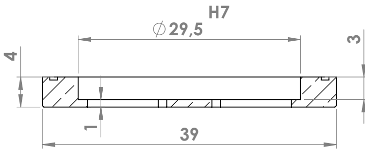
COUPE B-B
