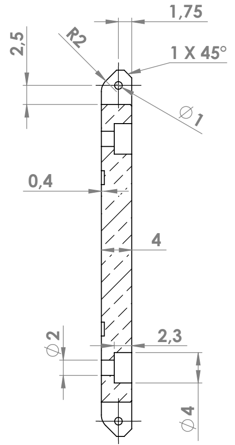
COUPE A-A
