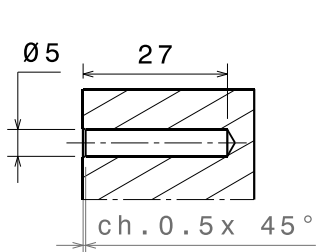
Coupe B-B Echelle : 1:1 Valable 5x
