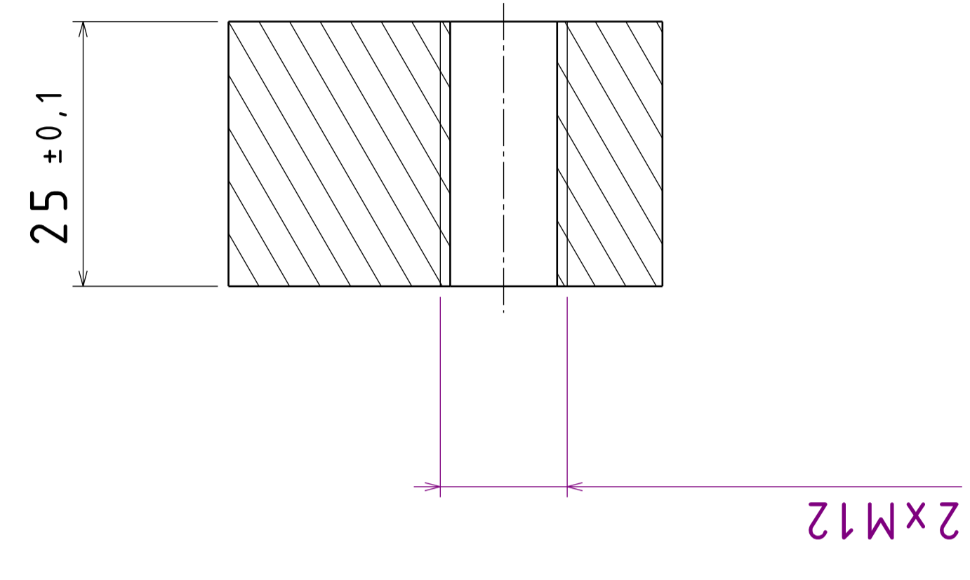
B-B Ech : 2:1
