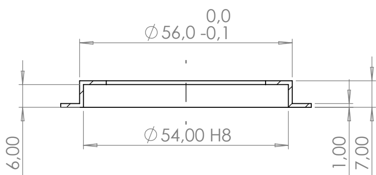
COUPE A-A
