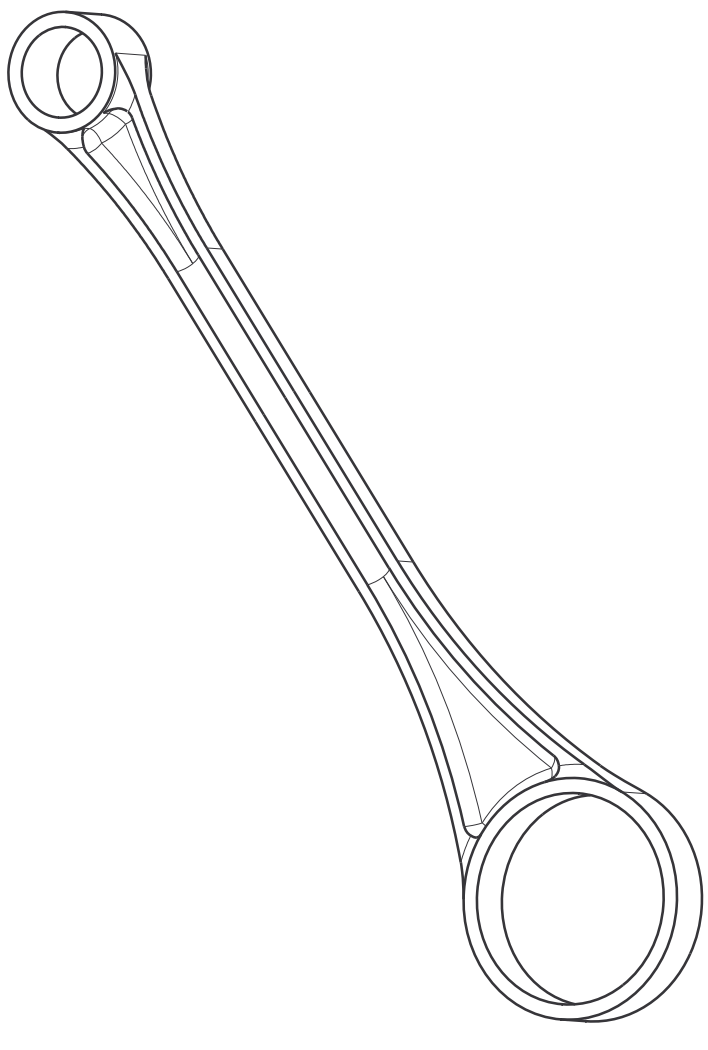
Vue isométrique Echelle : 1:1
