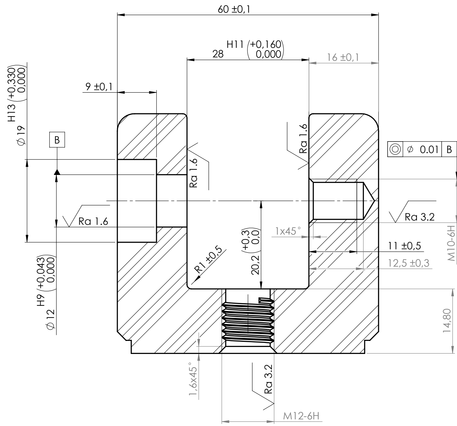
SECTION A-A
