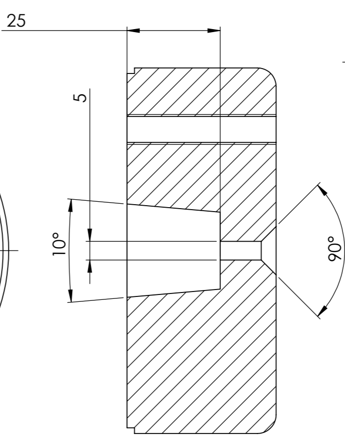
COUPE A-A
