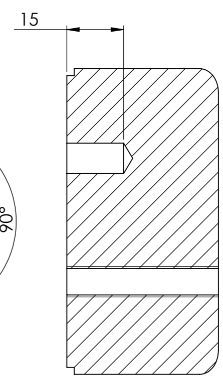
COUPE C-C
