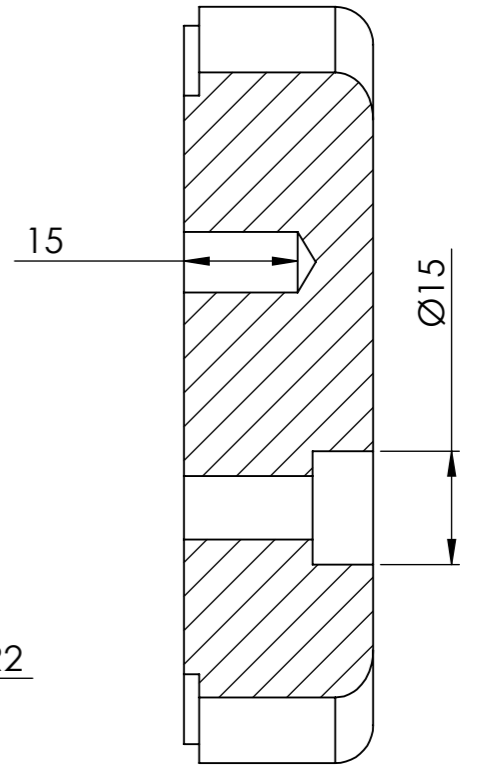
COUPE B-B
