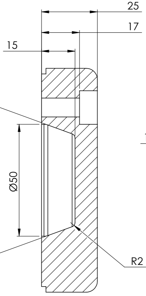
COUPE A-A
