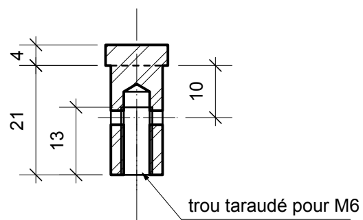
coupe BB
