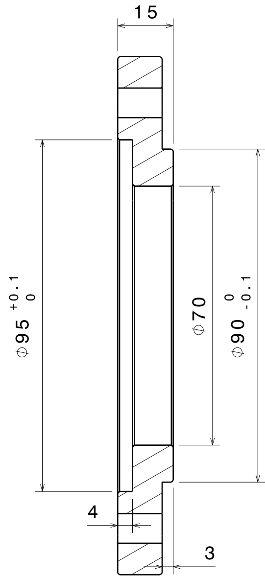
Coupe A-A Echelle : 1:1
