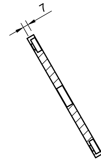
A-A (1:3)
