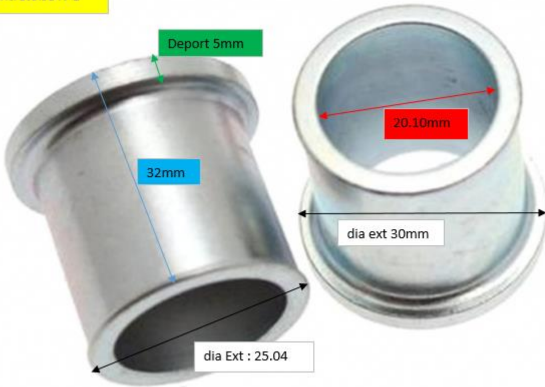
Entretoise N°2
