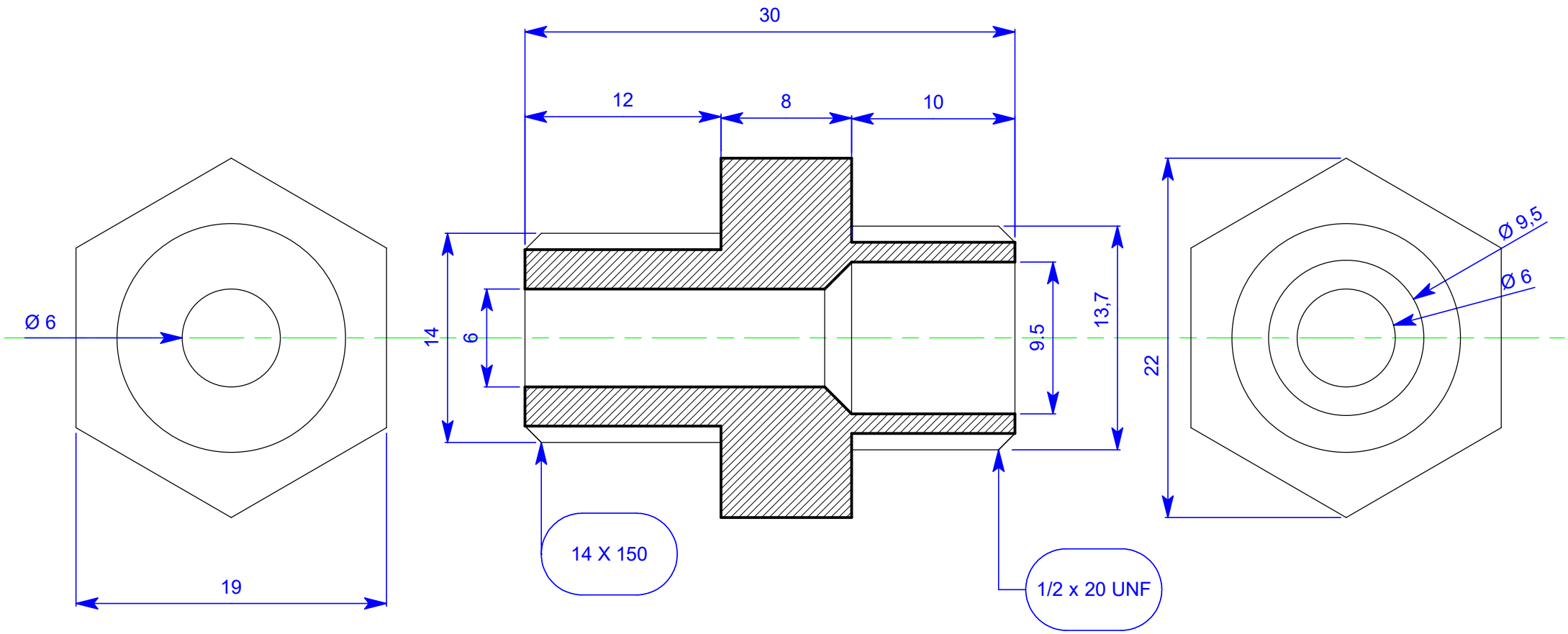
ELEVATION GAUCHE
