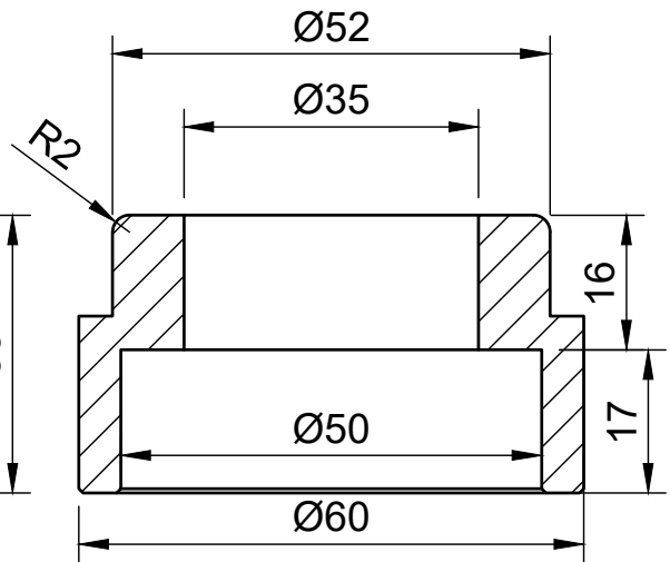
A-A (1:1)
