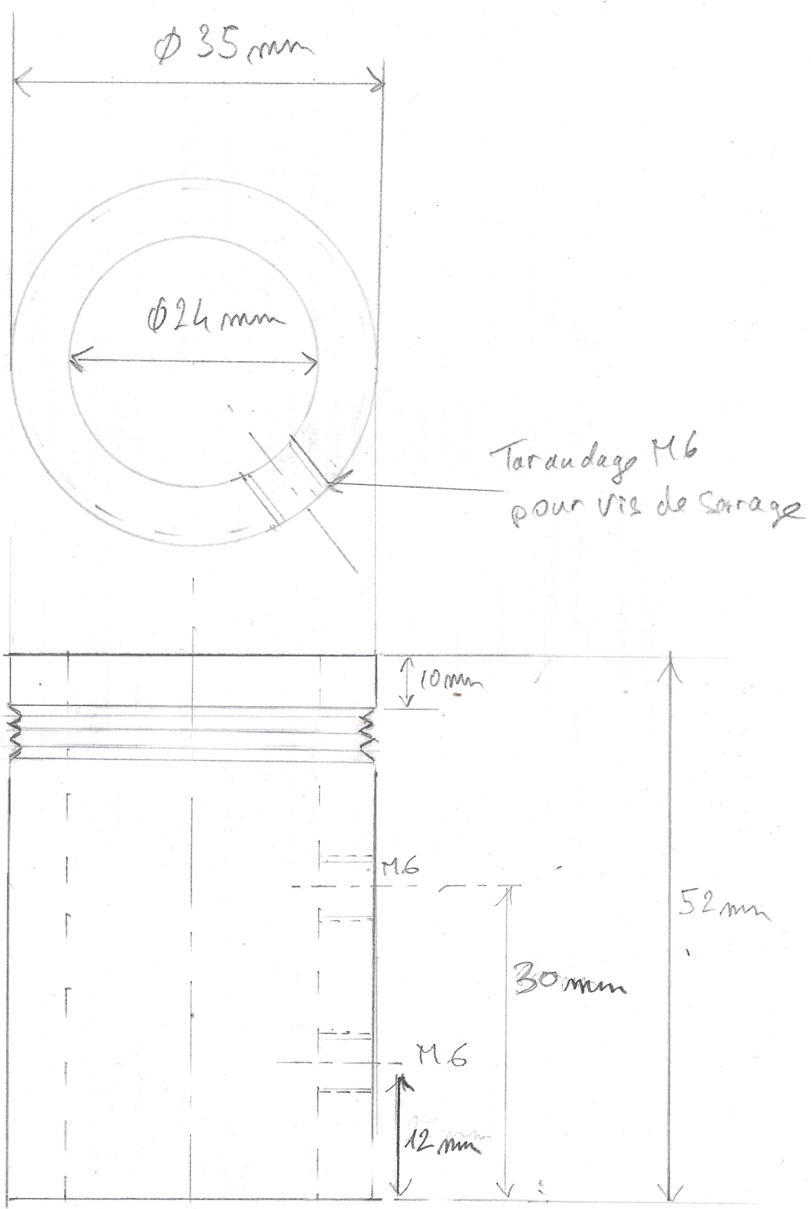
Poulie pour courroie Poly. V Aluminium
