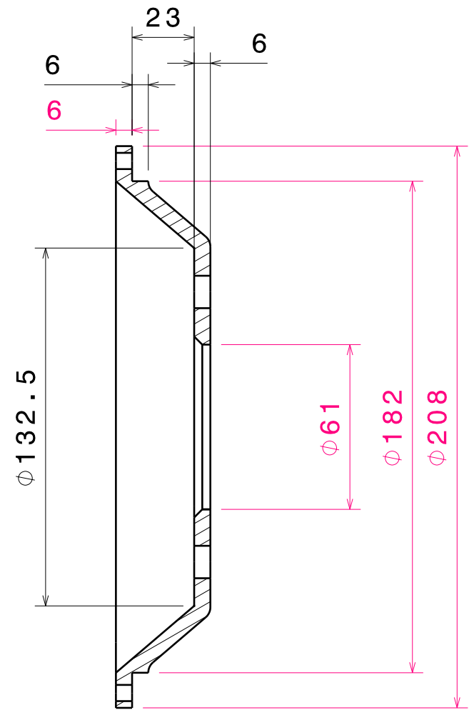
Coupe A-A Echelle : 1:2
