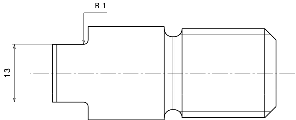
Top view Scale: 2:1
