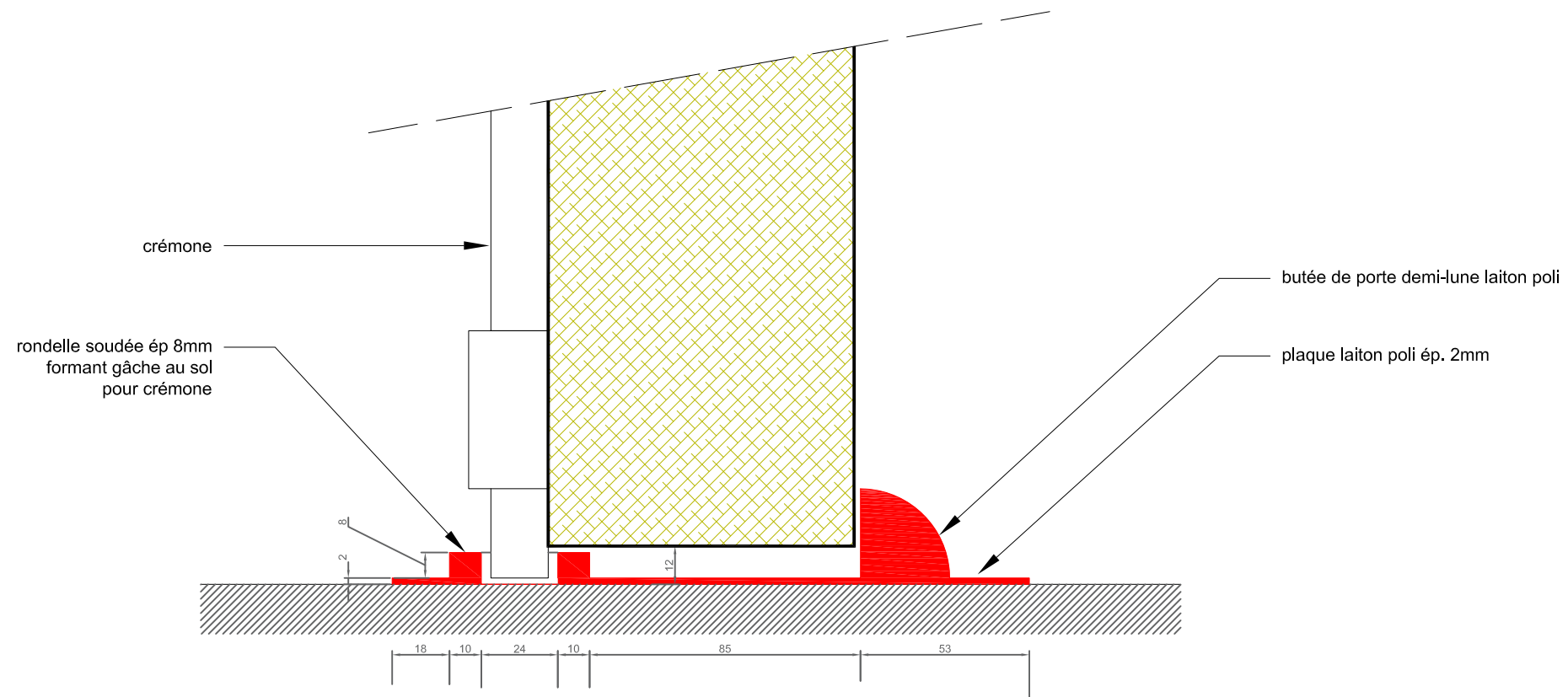
VUE EN COUPE
