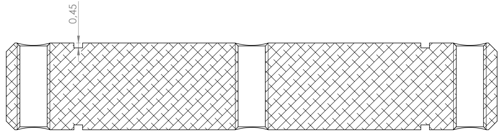
COUPE A-A
