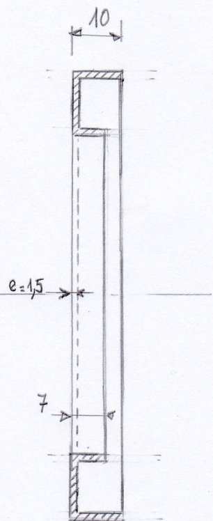
COUPE SUIVANT A-A
