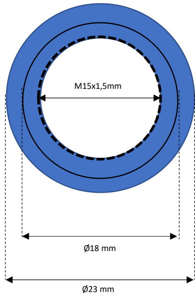
Coupe A-A
