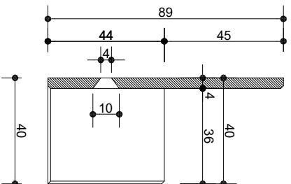
COUPE A-A
