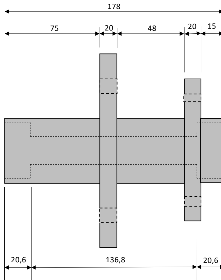
Vue coté
