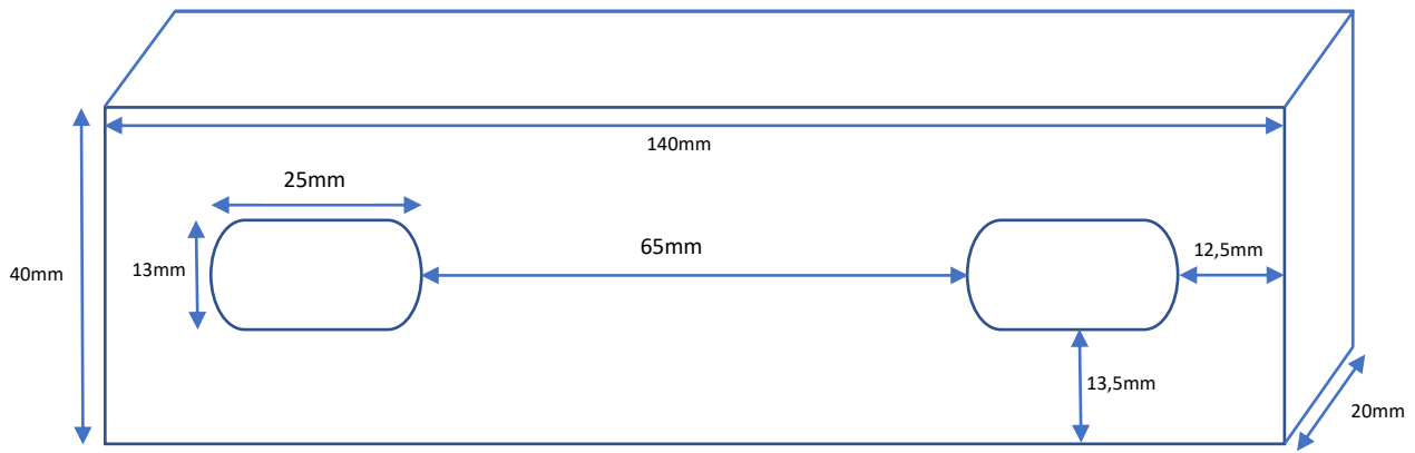
2 Entretoises en aluminium 140x40mm x épaisseur 20mm. Percées de 2 trous oblongs 25x13mm
