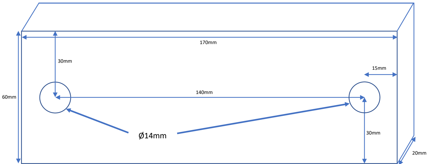
1 Entretoise en aluminium 170x60mm x épaisseur 20mm. Percées de 2 trous ronds \varnothing 14mm
