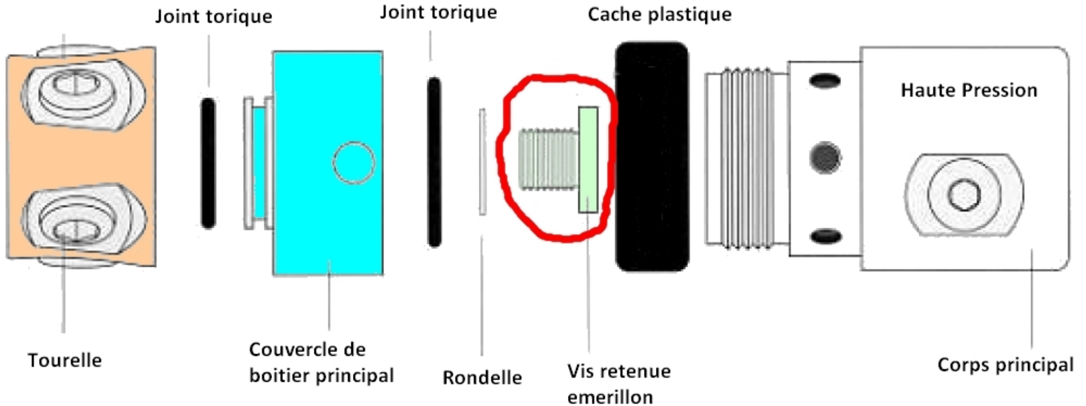
FIG.2 Liaison corps (tourelle)
