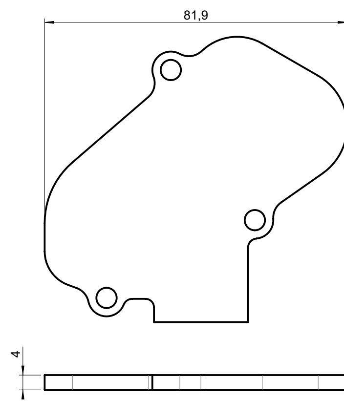
Acier S235 ou supérieur Quantité 1
