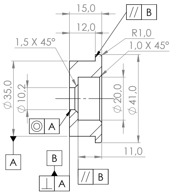
COUPE A-A
