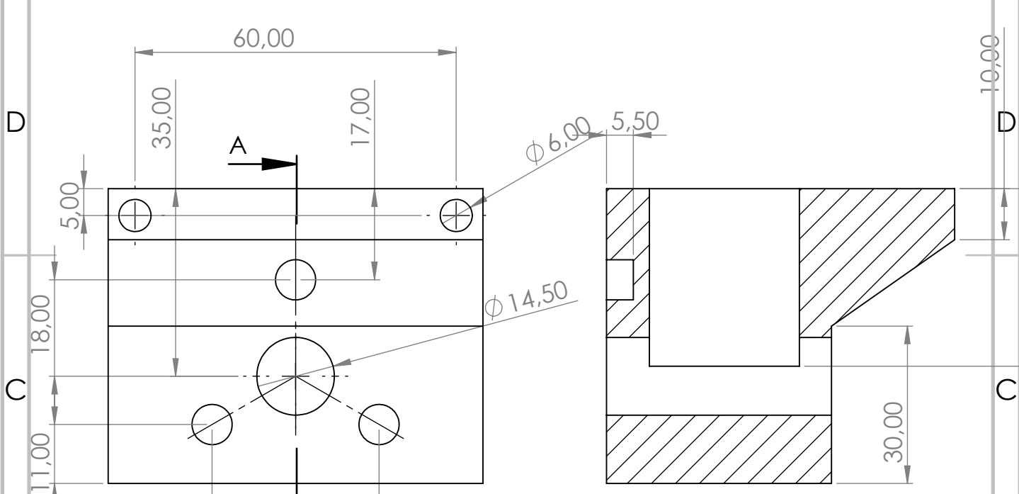
COUPE A-A ECHELLE 1 : 1
