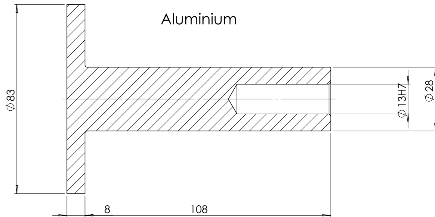
COUPE B-B
