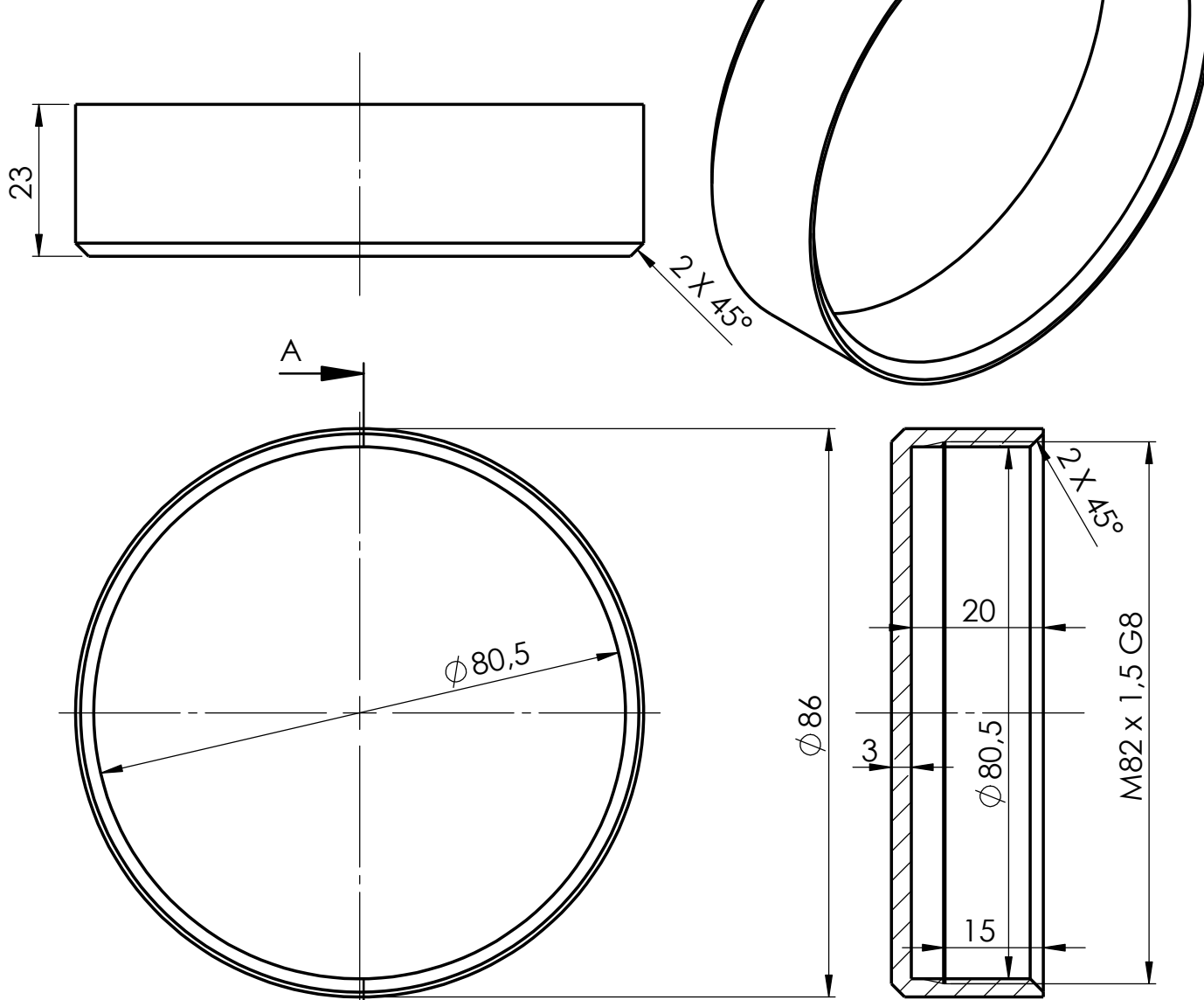
COUPE A-A
