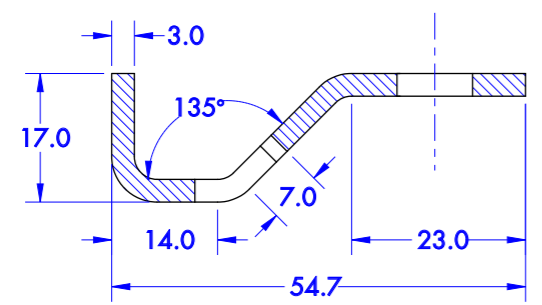
Coupe A-A
