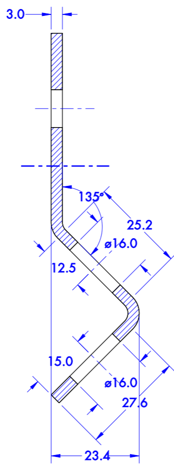
Coupe A-A
