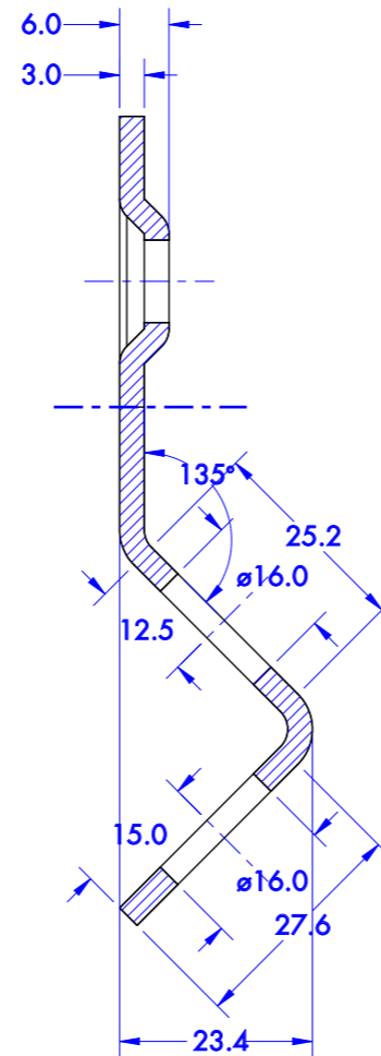
Coupe A-A
