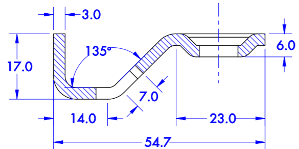
Coupe A-A
