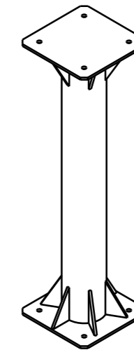
Vue isométrique Echelle : 1:20
