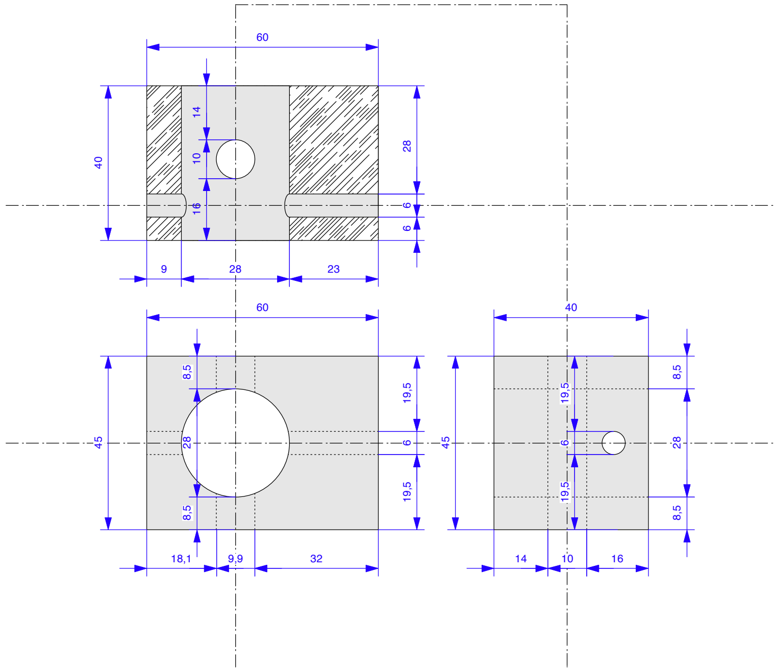
Parallélépipède rectangle en laiton percé de trois diamètres : Ø 28 mm / Ø 10 mm / Ø 6 mm
