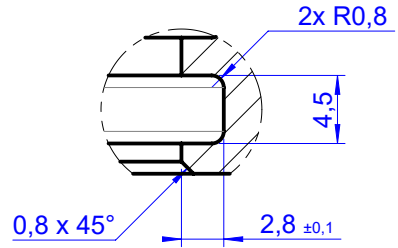
DÉTAIL B ECHELLE 2 : 1 2x gorges identiques
