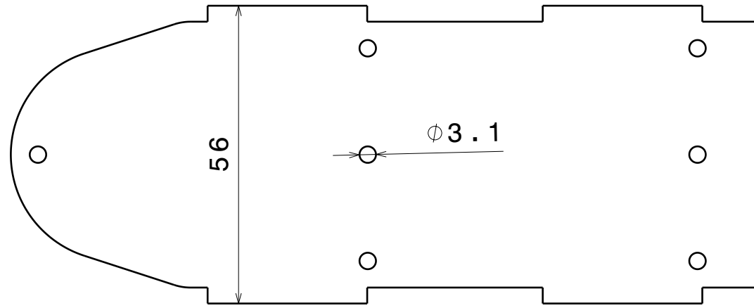
Vue de face Echelle : 1:1 PLATINE 2
