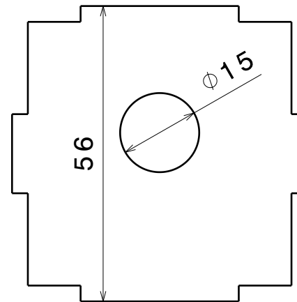
Vue de face Echelle : 1:1 PAROI 3
