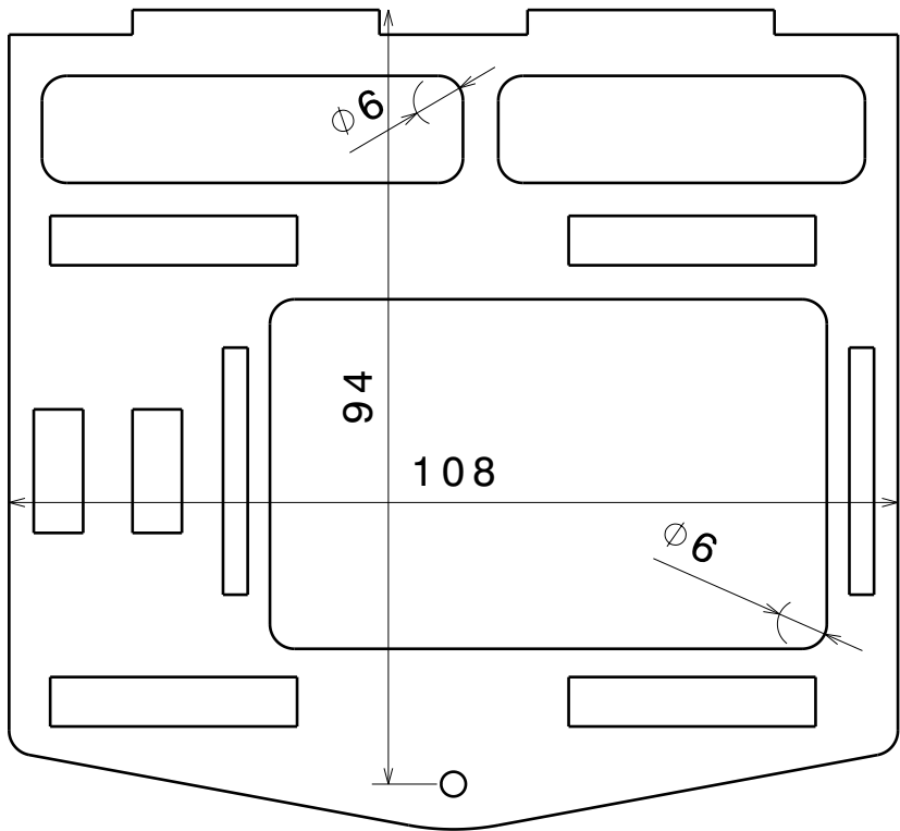
Vue de face Echelle : 1:1 PAROI 4
