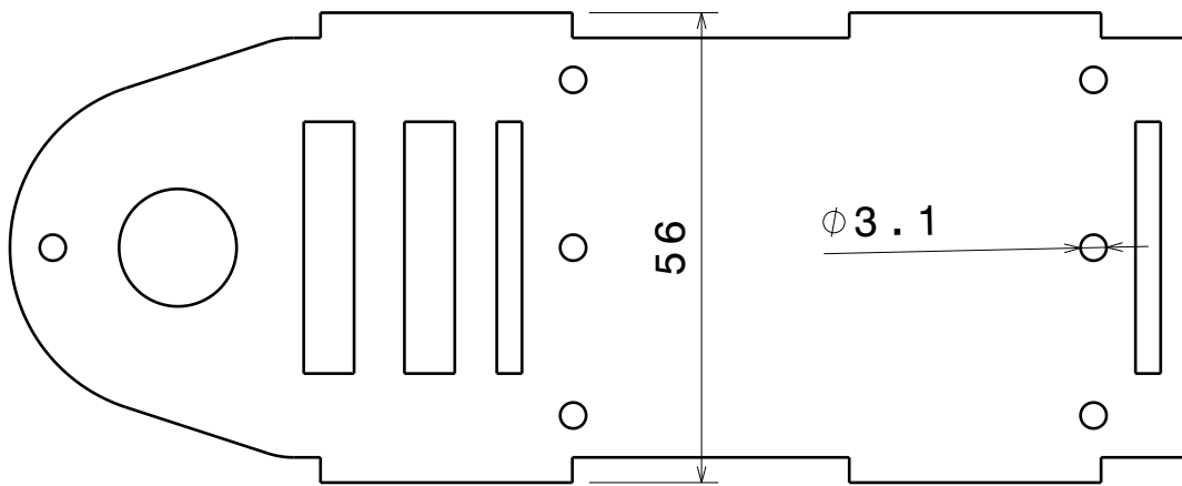
Vue de face Echelle : 1:1 PLATINE 1
