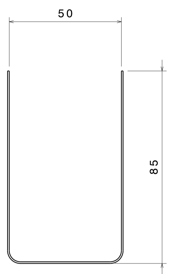
Vue de face Echelle : 1:1
