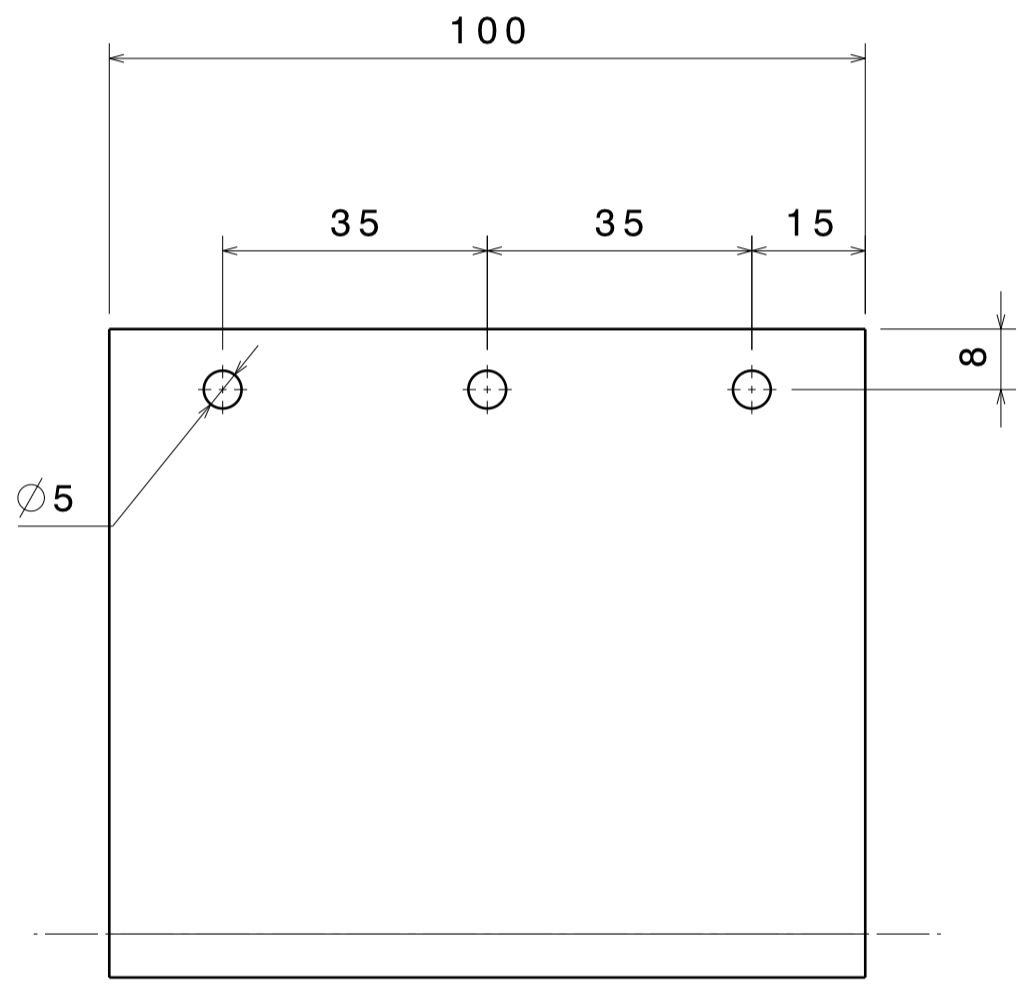
Vue de gauche Echelle : 1:1
