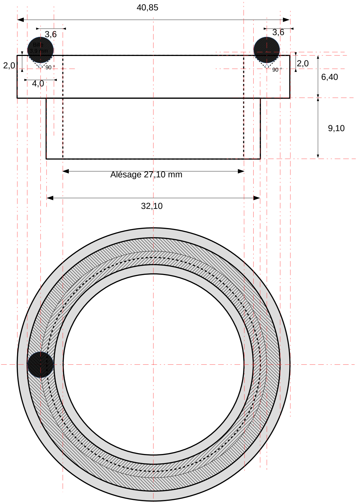
Butée externe de roulement à billes Acier 100CR6 cotes en mm
