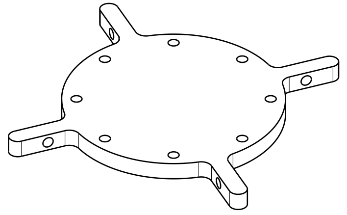
Vue isométrique Echelle : 1:1
