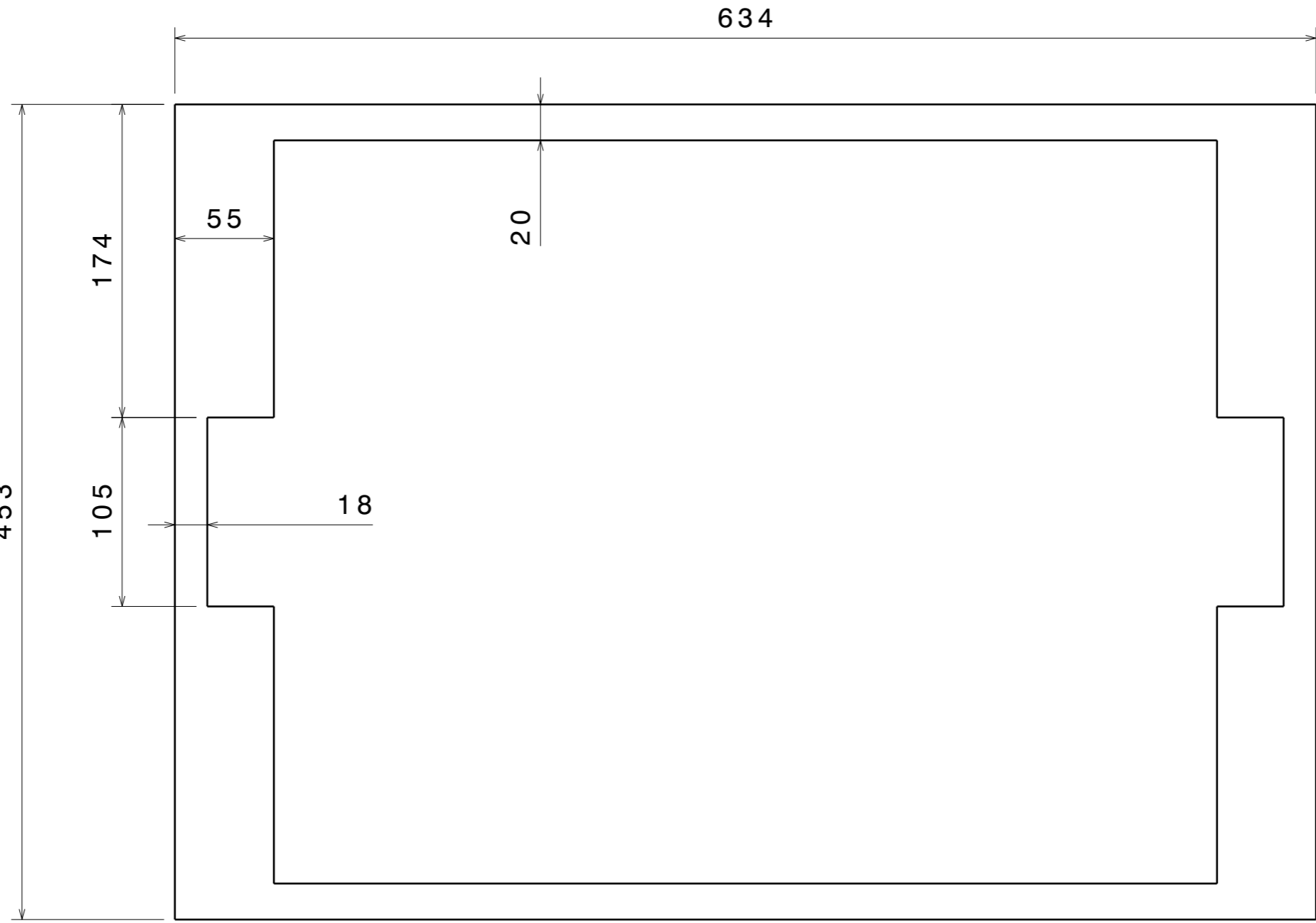
Vue de dessous Echelle : 1:3
